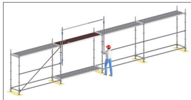
Rys. 35: Zastosowanie ochronnej poręczy wyprzedzającej w polu z przejściem
