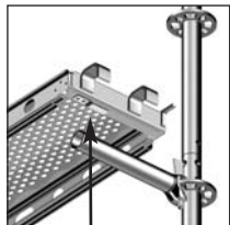
Rys. 12 zabezpieczenie przed podniesieniem
