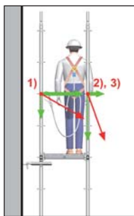
Rys. 27: Punkty zaczepienia na tarczy rozetowej (długość pola maksymalnie 3,07 m)
