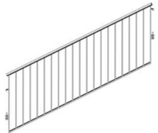
poręcz schodów 750, 8 stopni, nr art. 2638.101, 1,5 x 2,57 m
