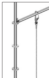
Rys. 30: Zaczepienie do 0-rygla
