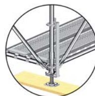
Ryc. 86: Mocowanie śruby przy pomocy zacisku klinowego
