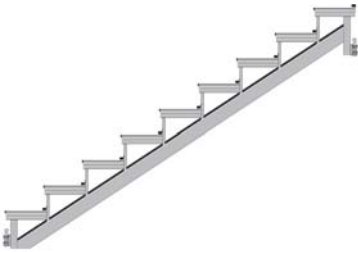
belka policzkowa schodów typu U 500, 9 stopni, nr art. 2638.009, 2,0 x 2,57 m
