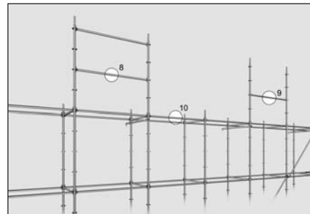
Rys. 29: Punkty zaczepienia do rygli Allround; długość pola maksymalnie 3,07 m
