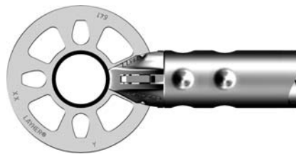
Rys. 3: Layher Allround aluminium według Z-8.22-64.1
